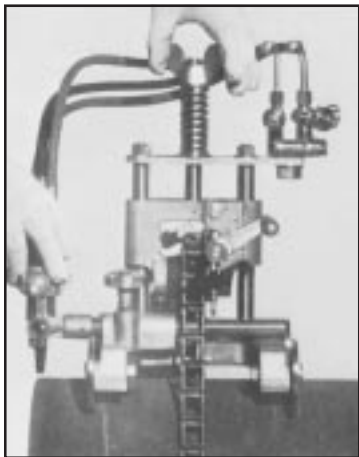
Corte perpendicular
